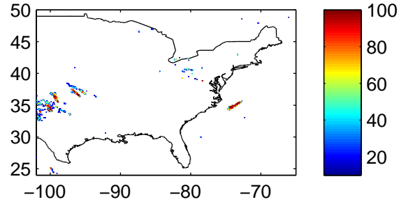
Max POSH 2012040912Z-2012041012Z
