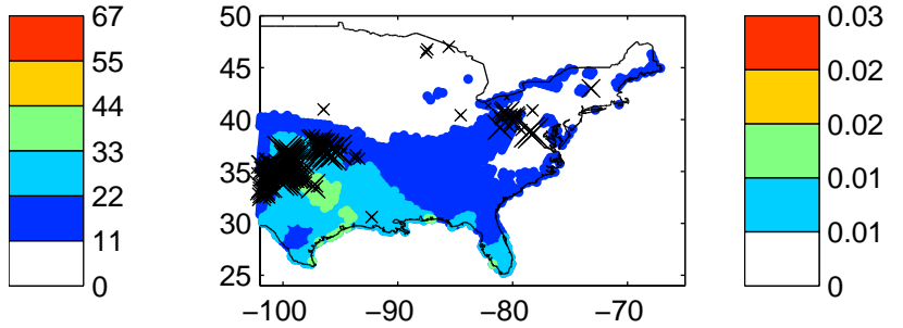
Max POSH 2012040912Z-2012041012Z
