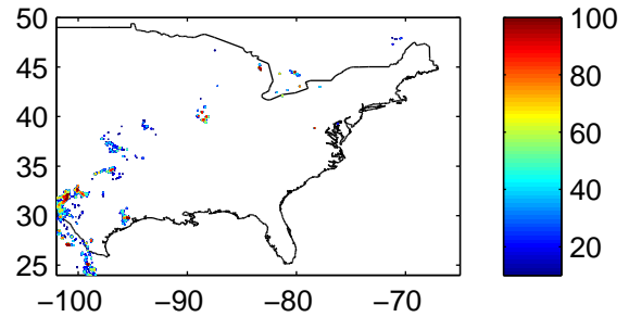
Max POSH 2012040712Z–2012040812Z
