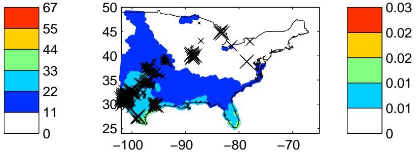
Max POSH 2012040712Z–2012040812Z
