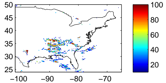
Max POSH 2012040512Z-2012040612Z
