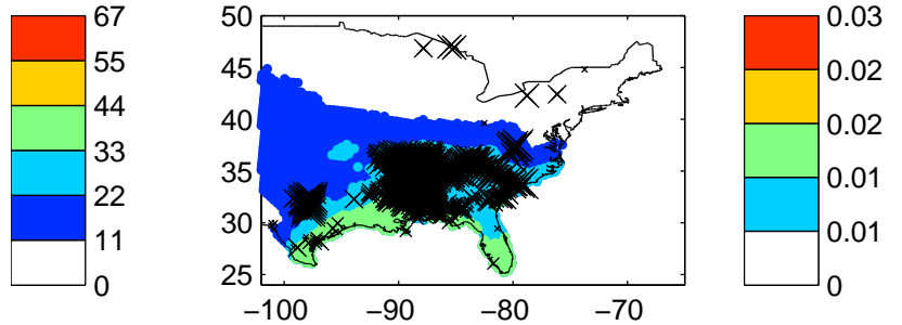
Max POSH 2012040512Z-2012040612Z
