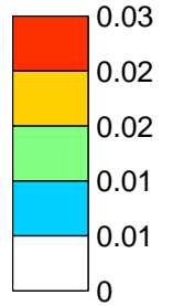
Surf hum (time max CAPE) 2012040412Z-2012040512Z
