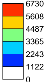
Surf hum (time max CAPE) 2012040412Z-2012040512Z
