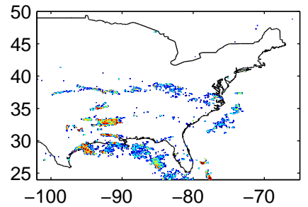
Max POSH 2012040412Z-2012040512Z
