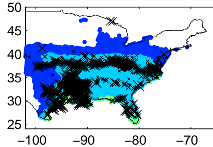
Max POSH 2012040412Z-2012040512Z
