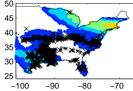
Surf hum (time max CAPE) 2012040412Z-2012040512Z
