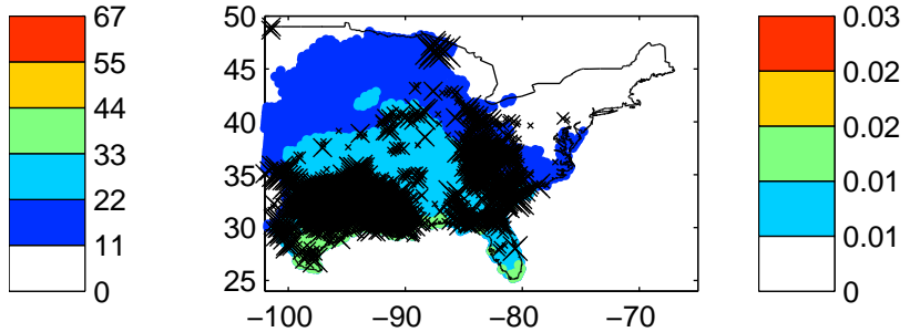
Max POSH 2012040312Z-2012040412Z
