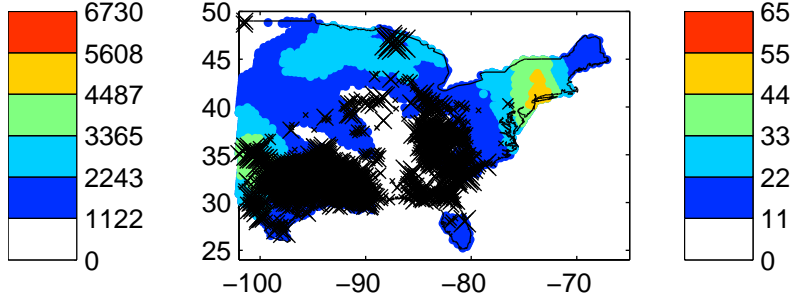
Surf hum (time max CAPE) 2012040312Z-2012040412Z
