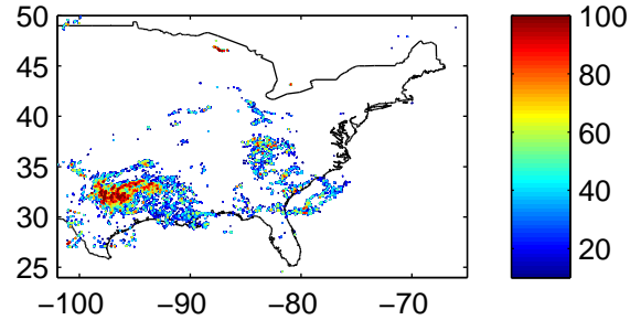
Max POSH 2012040312Z-2012040412Z
