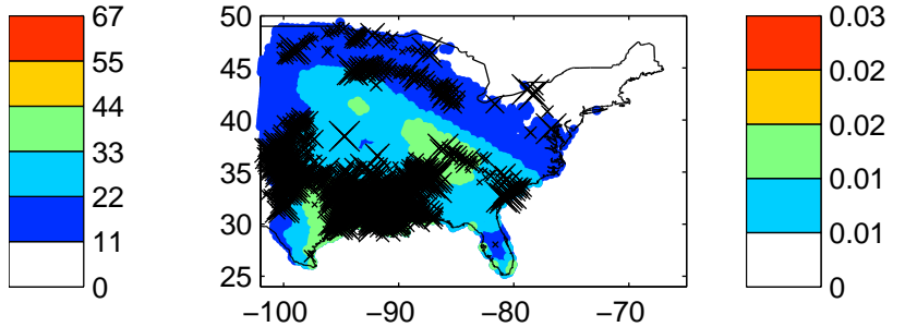
Max POSH 2012040212Z-2012040312Z
