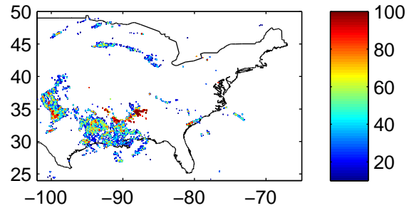
Max POSH 2012040212Z-2012040312Z
